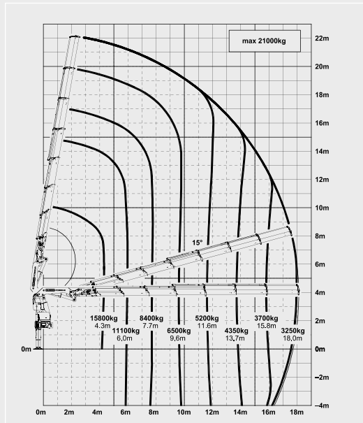
Lastdiagramm
